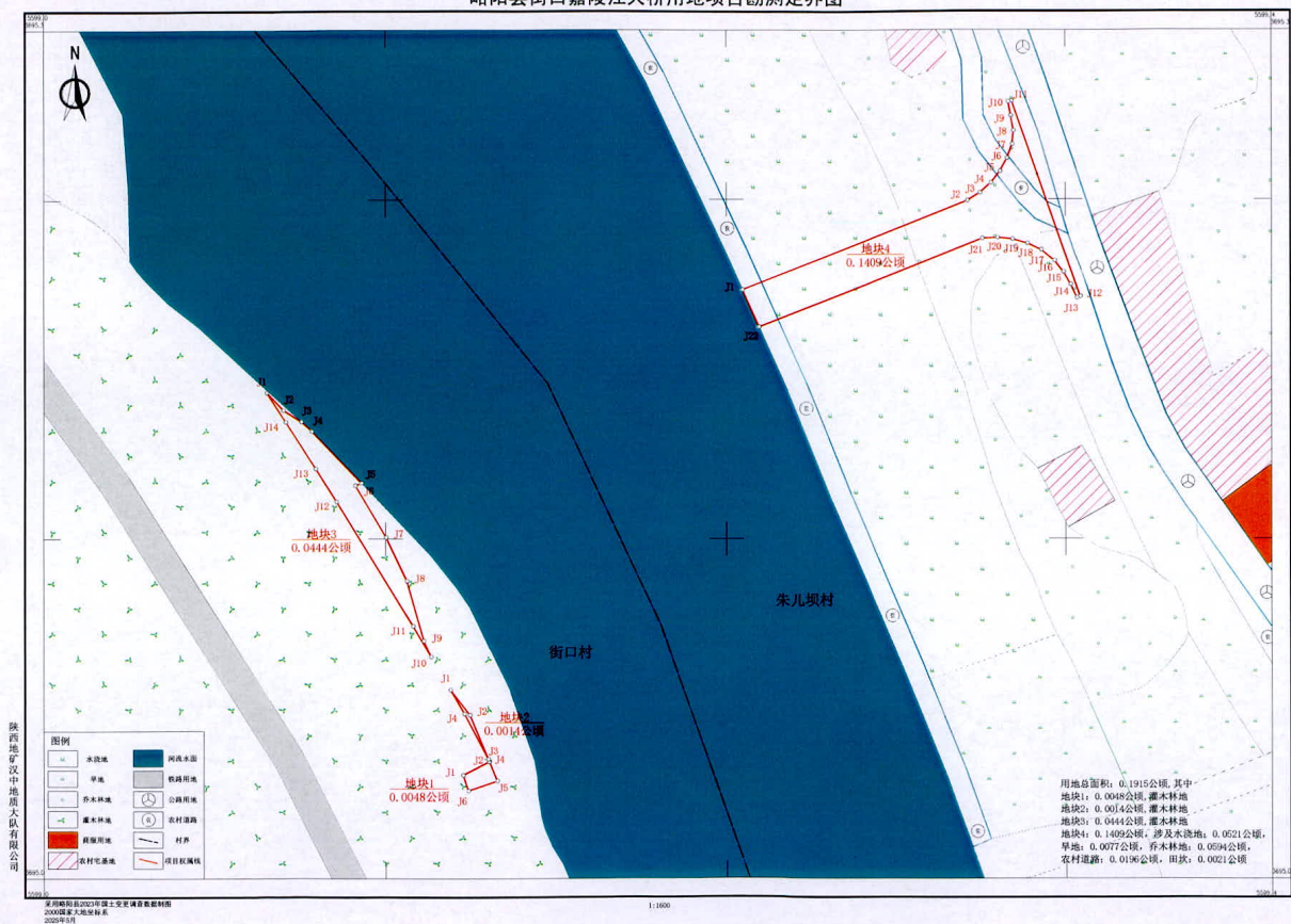
略阳县街口嘉陵江大桥用地项目勘测定界图
